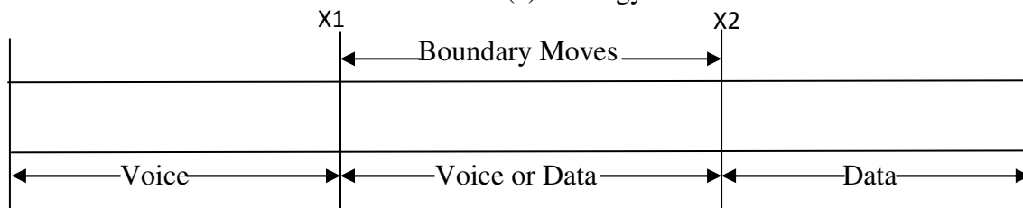
(d) Strategy 4
